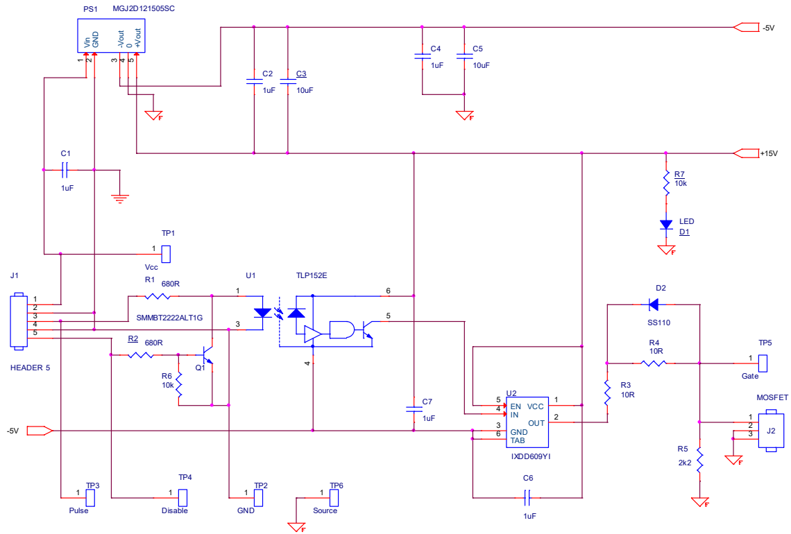
Fig.1. Esquema eléctrico del amplificador de compuerta Le-O4J15-09.
